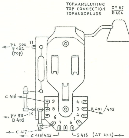
LIJNUITGANGS TRAFU LINE OUTPUT TRANSF. ZEILEN AUSG. ÜBERTRAGER AT 2023 50 051 709
